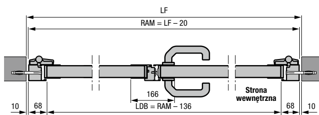
2-skrzydłowe drzwi boczne z aluminium ościeżnicą blokową, profil typu 2 Montaż w otworze
