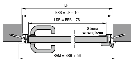
Drzwi boczne z aluminium ościeżnicą kątową, profil typu 2 Mocowane od wewnątrz
