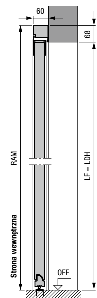
Drzwi boczne z aluminium ościeżnicą blokową, profil typu 2 Montaż za otworem
