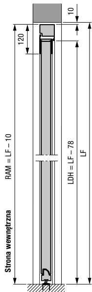
Drzwi boczne z aluminium ościeżnicą blokową, profil typu 2 Montaż w otworze
