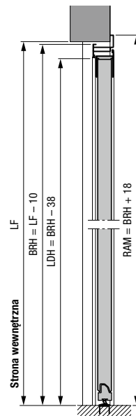
Drzwi boczne z aluminium ościeżnicą kątową, profil typu 2 Mocowanie od zewnątrz
