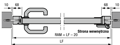
Drzwi boczne z aluminium ościeżnicą blokową, profil typu 2 Montaż w otworze
